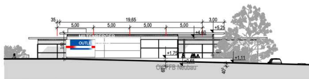
Ansicht Osten
