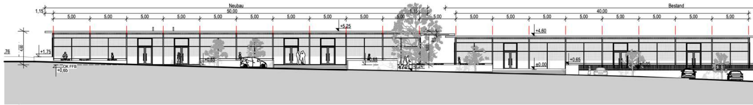
Ansicht Norden
